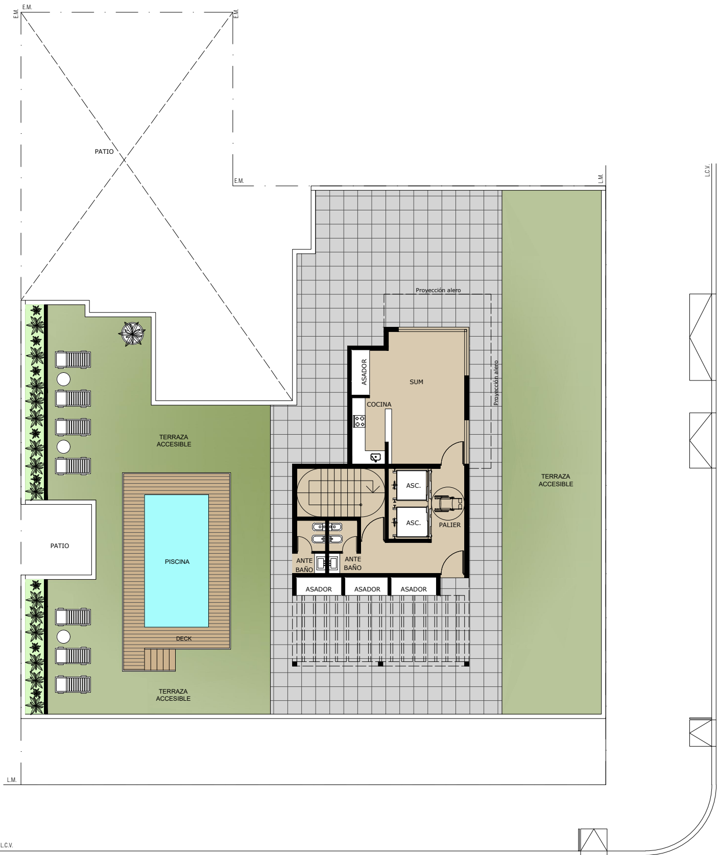
PLANTA DE AZOTEA, ESC. 1:100
